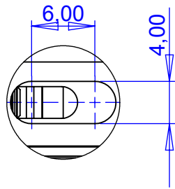
DÉTAIL B ECHELLE 2 : 1
