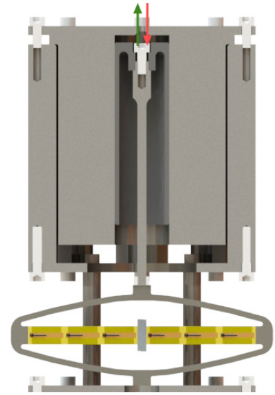
Fig. 7 : Piezo PWG/SJA principle
