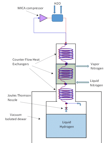
Fig. 14 : Schema principle
