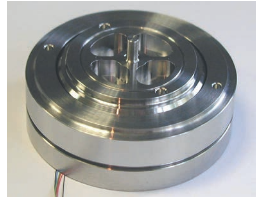
Fig. 1.a: RPA motor
