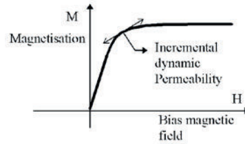
Fig. 2: M(H) curve.
